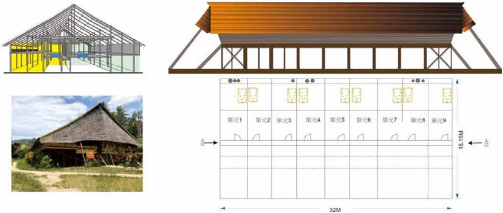
圖16 長屋外觀與架構圖
