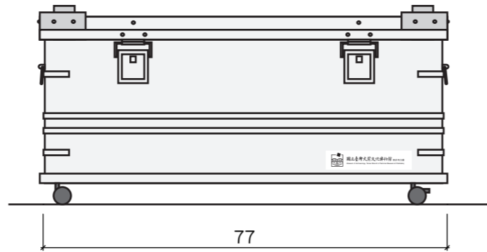
立面圖
