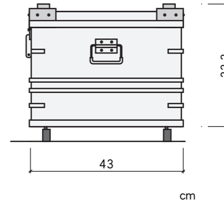
側立面圖
